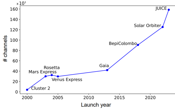
Figura 1: Evolución a través de los años de la cantidad de variables para diferentes misiones de la ESA [2].
