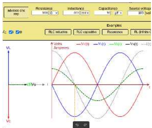
Figura 3: Interfaz web mostrando el diagrama fasorial de un circuito RLC en resonancia
