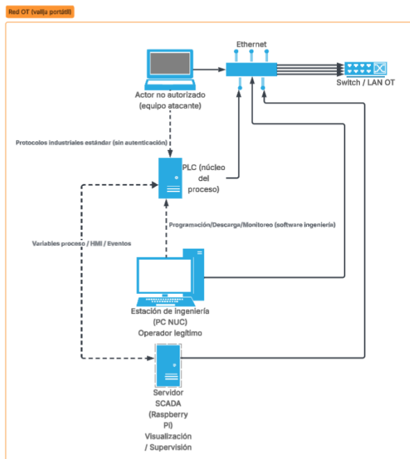
Figura 1. Topología de red OT del banco de pruebas portátil.
