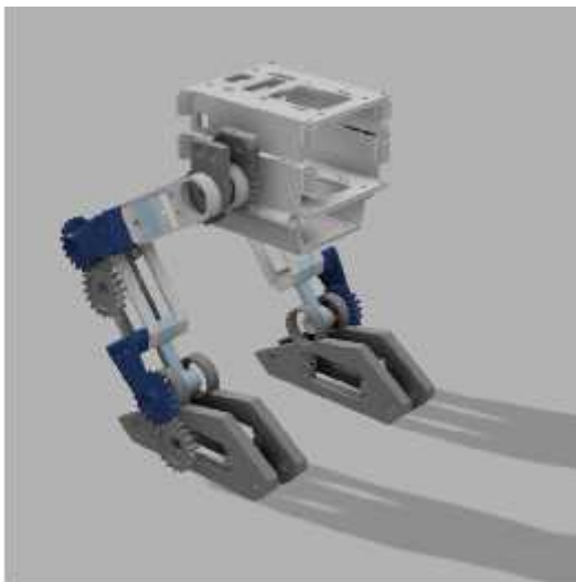
Fig 1. Modelo CAD completo ensamblado en Fusion 360.
