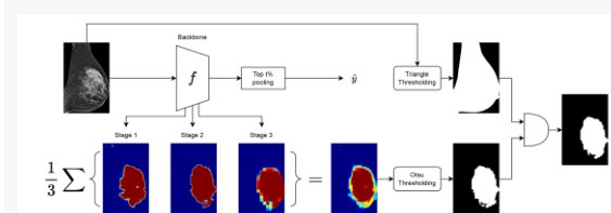
Figura 4. Método propuesto de generación de segmentaciones con etiquetas débiles. Se entrena un clasificador con etiquetas generales de clase (A vs D de la clasificación BI-RADS). Luego se generan máscaras mediante GradCAM, que se utilizan como etiquetas débiles para entrenar un modelo de segmentación.
