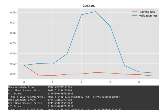
Figura 4: Gráfica de error RNN - Fuente: elaboración propia
