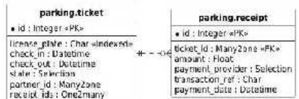
Figura 1: Modelo de Datos (Extensión de Odoo)
