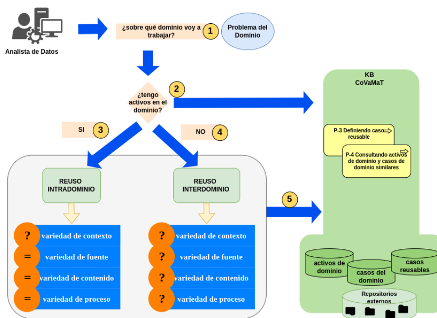
Figura 3: Proceso para reutilizar utilizando CoVaMaT
