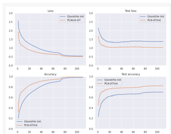
Figura 3. Los filtros de un modelo ViT inicializados mediante el método propuesto mejoran la velocidad de convergencia en algunos escenarios
