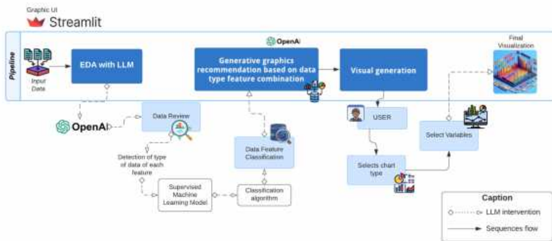
FIGURA 1. Arquitectura de VisBot: 1) EDA con LLM; 2) recomendación de gráficos generativos basada en la combinación de características del tipo de datos; y 3) generación visual y mejoras adicionales; 4) visualización final generada.
