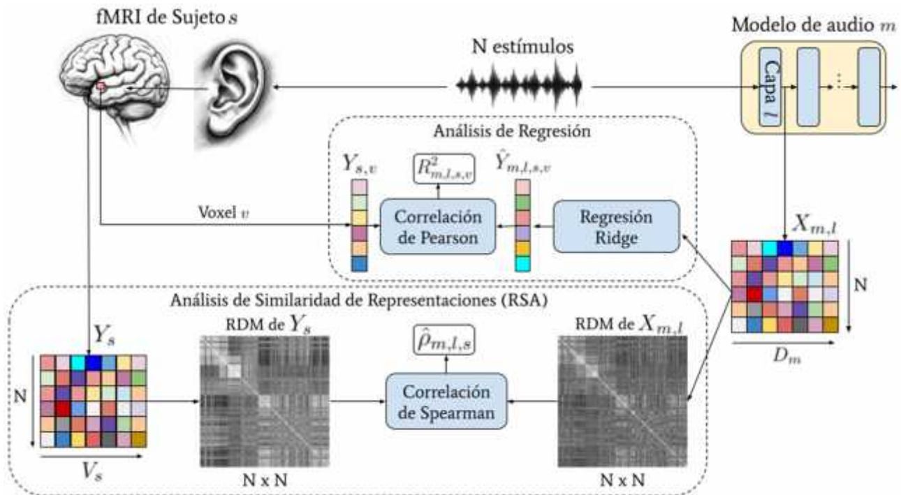
Figura 3. Diagrama resumen de la metodología utilizada para comparar las representaciones de audio con las mediciones de fMRI.
