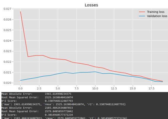
Figura 4: Gráfica de error GRU - Fuente: elaboración propia
