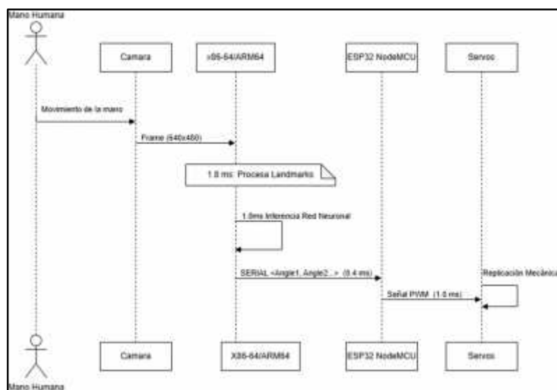
Figura 1. Diagrama de secuencia del flujo de datos. Se observa la distribución de carga entre la unidad de alto desempeño (PC) y el controlador de periféricos (ESP32), logrando un tiempo de respuesta end-to-end de 4.2 ms.
