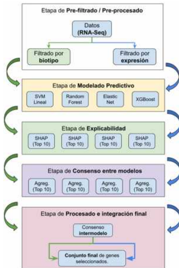
Figura 1: Representación visual del pipeline propuesto.
