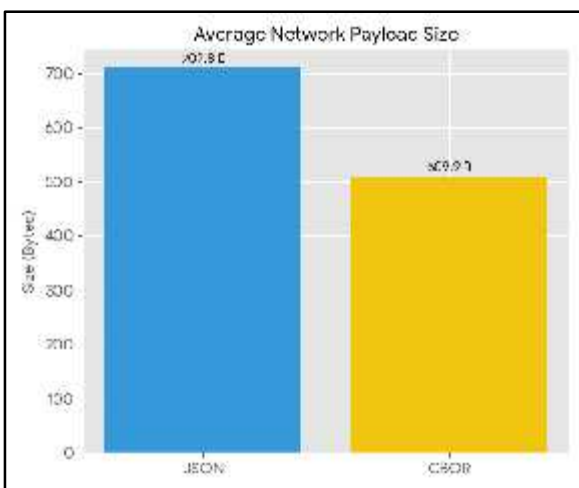
Fig. 2. Reducción relativa del tamaño de la carga útil lograda por CBOR en la transmisión IIoT.
