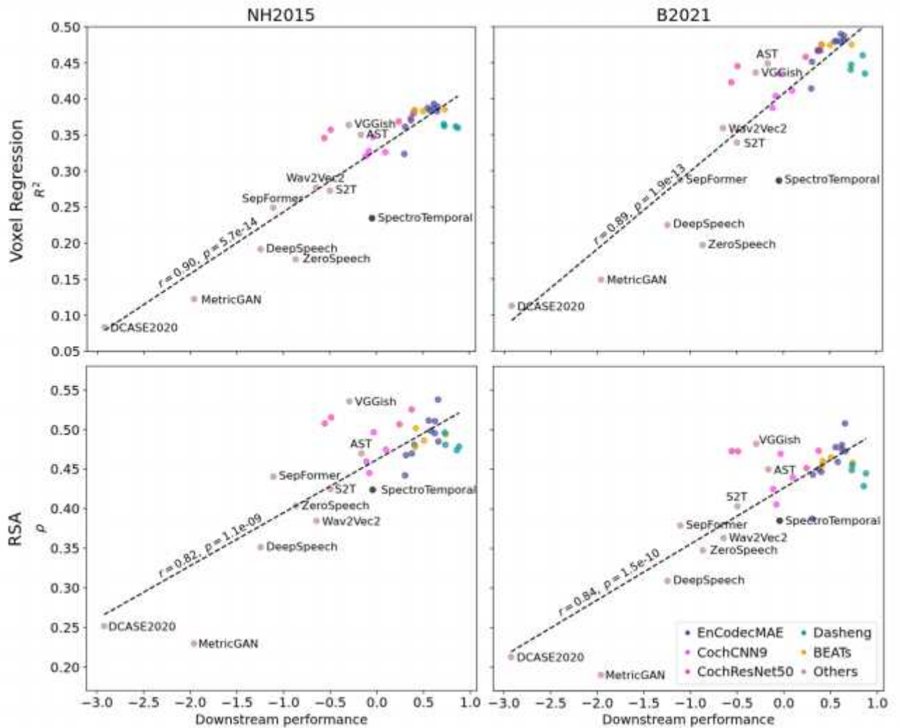
Figura 4. Gráficos de dispersión comparando el desempeño promedio normalizado de cada modelo de audio con su similaridad con las mediciones de fMRI, para ambos conjuntos de datos, y obtenidas tanto mediante RSA como regresión ridge.
