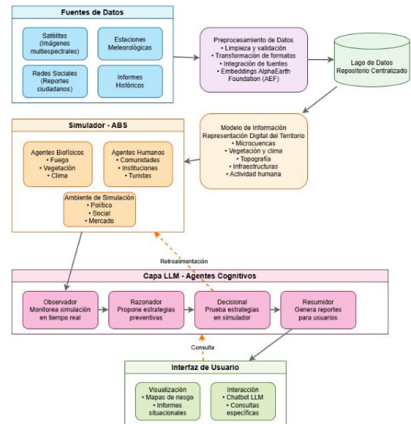
Figura 1: Arquitectura del gemelo digital.
