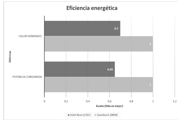
Figura 2. Comparación de eficiencia energética entre arquitecturas CISC y RISC.
