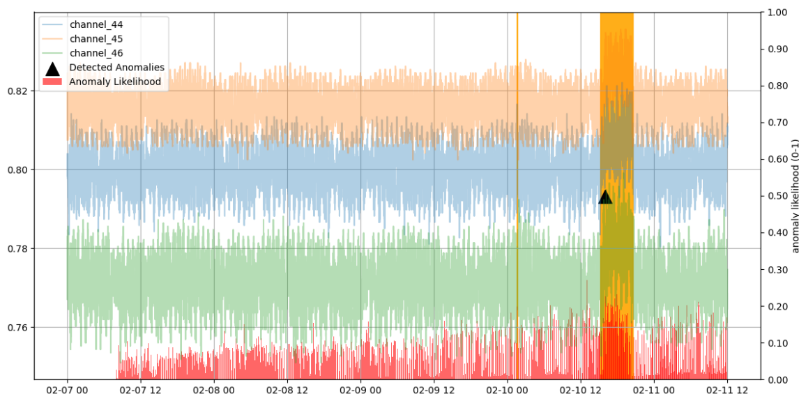
Figura 4: HTM[9] aplicado a los canales 44, 45 y 46 del dataset de la ESA [13] mostrando capacidad de predicción de anomalías multicanal. Es sector sombreado representa las anomalías etiquetadas por la ESA. Las barras rojas al pie muestran la propensión de anomalías detectadas por el modelo y los triángulos lugares donde se supera un umbral predefinido a partir de ensayos.
