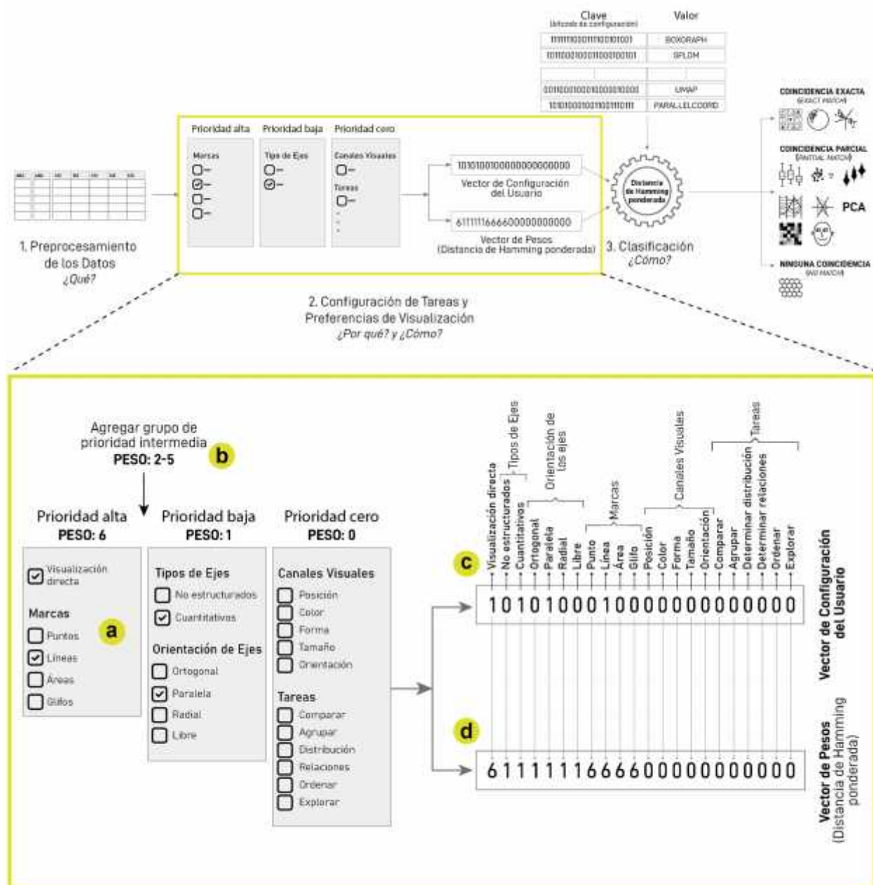
Figura 3: Arquitectura del sistema CVRS. (1) Pre procesamiento de los datos: se clasifican los datos en categóricos y numéricos, permitiendo al usuario seleccionar las columnas clave para su visualización. (2) Configuración de tareas y preferencias de visualización: el usuario define los parámetros que orientarán la visualización de los datos de acuerdo con sus preferencias de representación visual y objetivos de análisis. (3) Clasificación: el sistema selecciona las técnicas de visualización más adecuadas para comunicar de manera efectiva la información.
