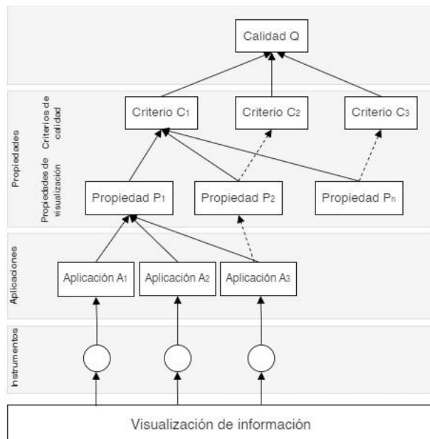
Fig. 2: Elementos y estructura del metamodelo.
