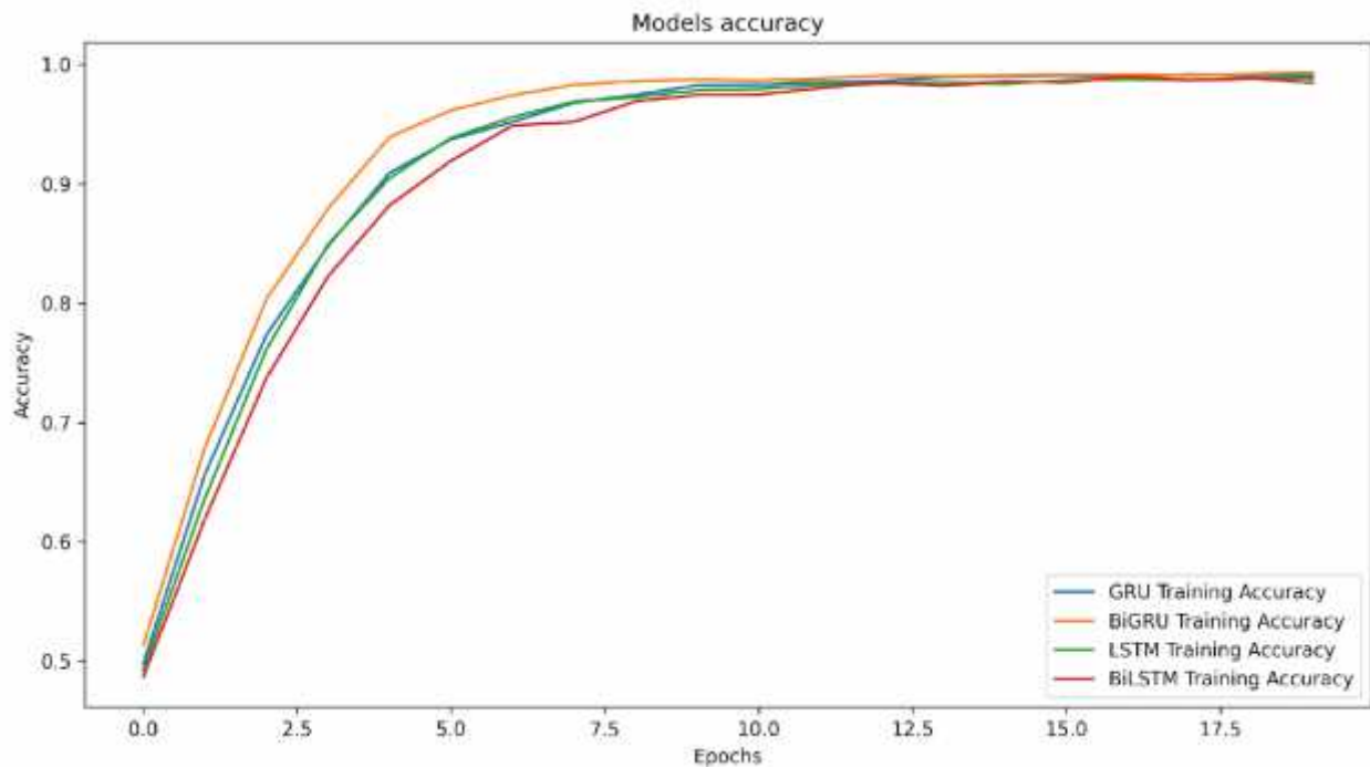
Figura 3. Comparación de la exactitud de los algoritmos.
