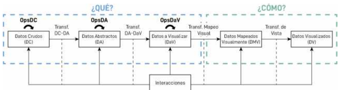
Figura 1: Modelo Unificado de Análisis Visual (UVAM) presentado por Ganuza et al. en el contexto de los tres pilares de la visualización. Figura adaptada de [GULC23].
