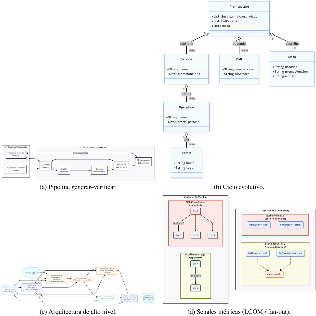
Figura 1: Resumen visual de ArchiGenMS: flujo general, búsqueda evolutiva, arquitectura de orquestación e intuición de métricas.
