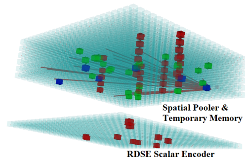
Figura 2: Representación conceptual del codificador, en este caso un codificador RDSE junto con un Spatial-Pooler y un TemporaryMemory en la sección superior. El color rojo indica una neurona activa, el azul una neurona predictiva y el verde una neurona ganadora. Se presenta una versión simplificada de alto nivel de un modelo HTM[9] con fines ilustrativos; la topología real, el total de neuronas y la cantidad de neuronas por columna puede variar respecto a esta esquematización. La figura es de generación propia utilizando la biblioteca pyvista[10].
