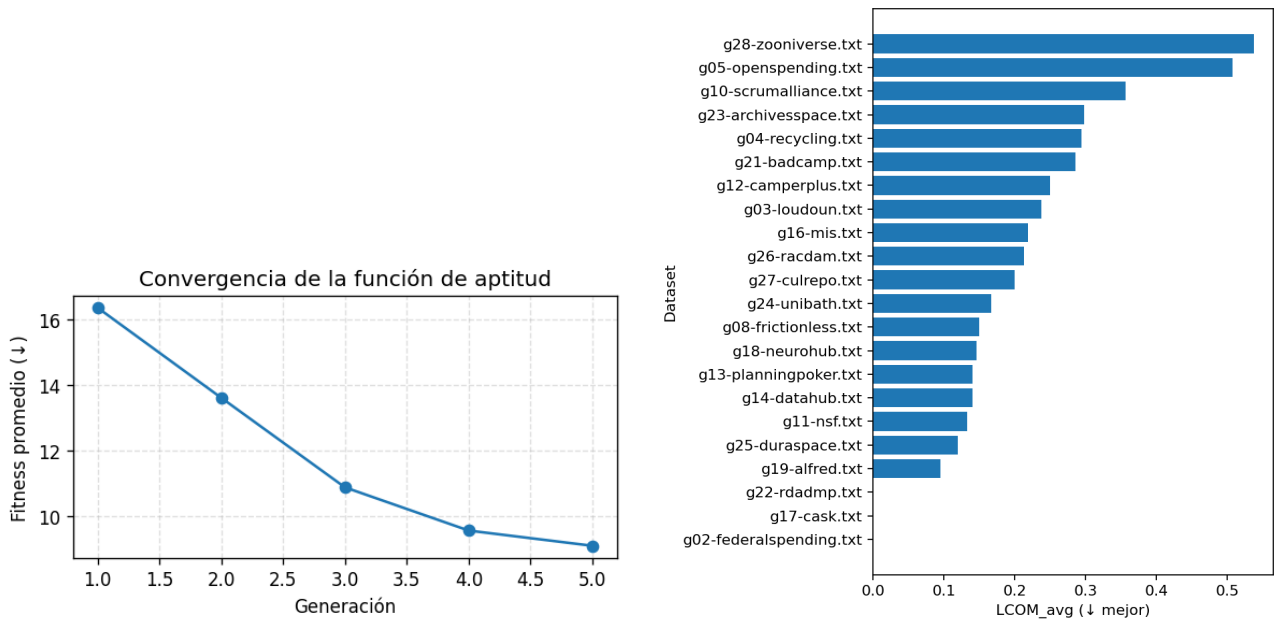
Figura 2: Evidencia empírica: convergencia agregada y heterogeneidad por escenario.
