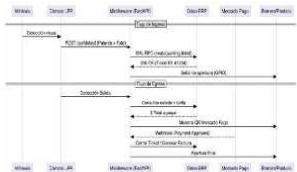
Figura 2: Diagrama de secuencia del ingreso y egreso de vehículos
