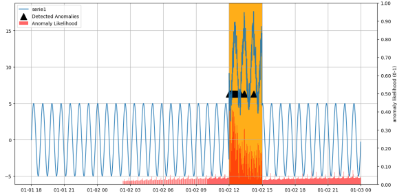
Figura 3: HTM[9] aplicado a una señal senoidal. Es sector sombreado representa las anomalías artificialmente generadas. Las barras muestran la propensión a una anomalías detectada por el modelo y los triángulos lugares donde se supera un umbral predefinido.
