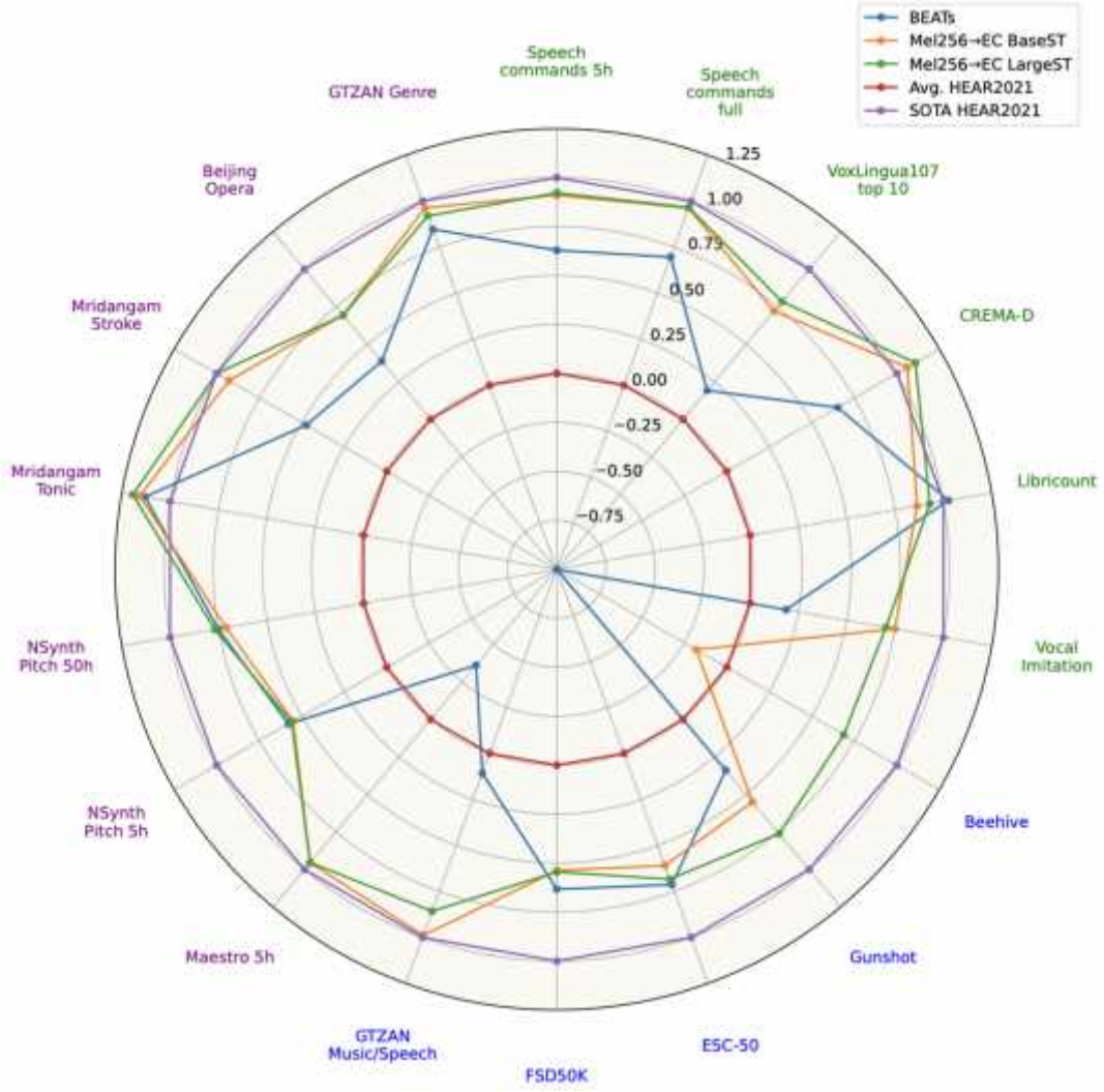
Figura 2. Desempeño normalizado de los modelos propuestos contra el estado del arte.
