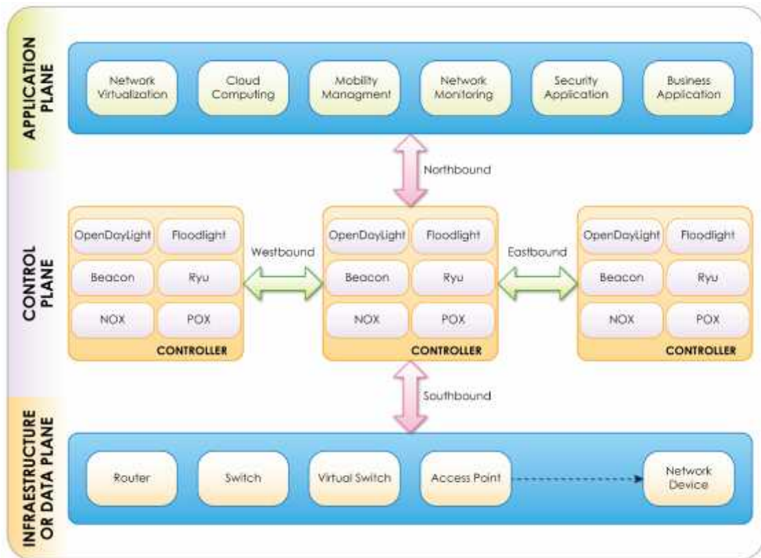
Figura 1. Arquitectura de redes definidas por software.
