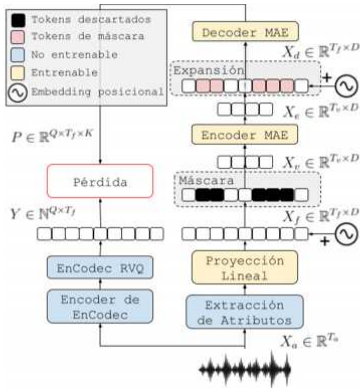
Figura 1. Arquitectura de EnCodecMAE
