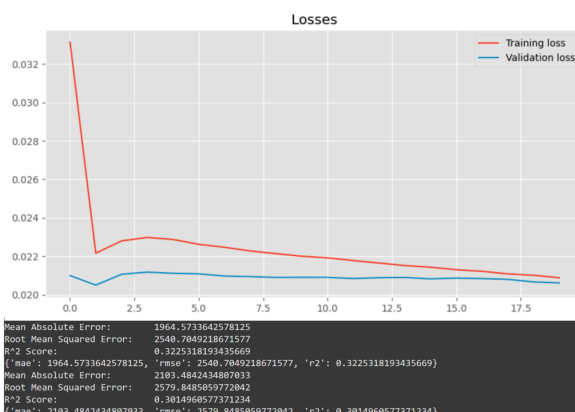
Figura 3: Gráfica de error LSTM - Fuente: elaboración propia
